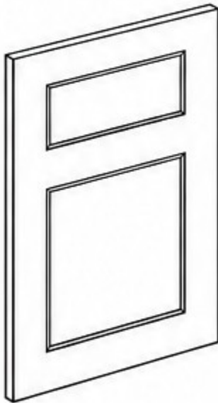
Example shown: 715 × 496 mm door
